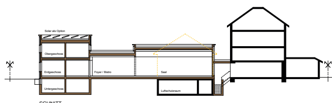
Querschnitt
